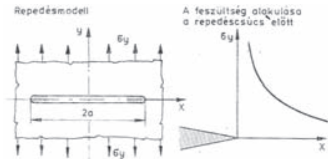
1. ábra Repedésmodell és feszültségkoncentráció Griffith szerint [8] Fig. 1. Crack model and stress concentration according to Griffith [8]
