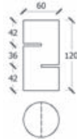
17. ábra Félbevágott, 60 mm átmérőjű henger elvi kialakítása Fig. 17. Schematic shape of a half notched cylinder, diameter 60 mm
