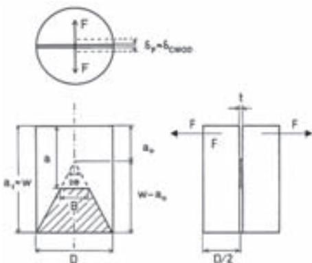
6. ábra „Negatív V” bemetszésű próbatest (Short Rod) [16] Fig. 6. Specimen (Short Rod) with „negative V” notch [16]
