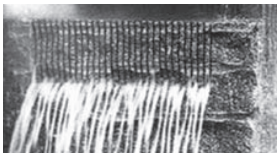
Fig. 2. Cutting the block in plates 2. ábra Kőtömbök lapokra fűrészelése
