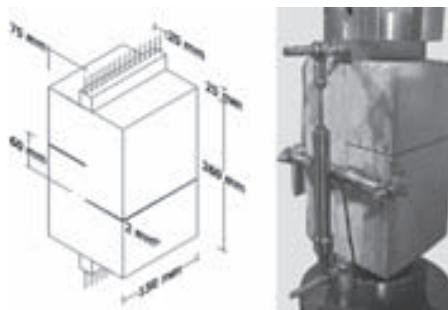
9. ábra Félig-félig bemetszett próbatest nyíróvizsgálata [19] Fig. 9. Shear test of a half-half notched specimen [19]
