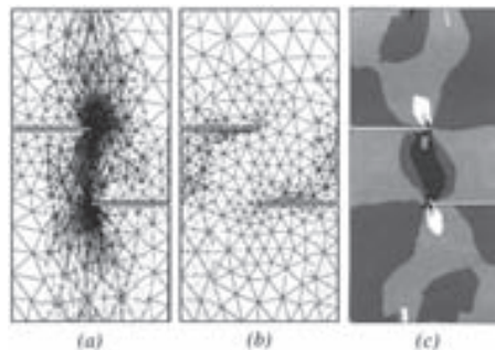
10. ábra Nyíróvizsgálat végelelemes modellezése (a) nyomófeszültség; b) húzófeszültség; c) nyírófeszültség eloszlása) [19] Fig. 10. FE modelling of shear test (a) compressive stress; b) tension stress; c) shear stress) [19]
